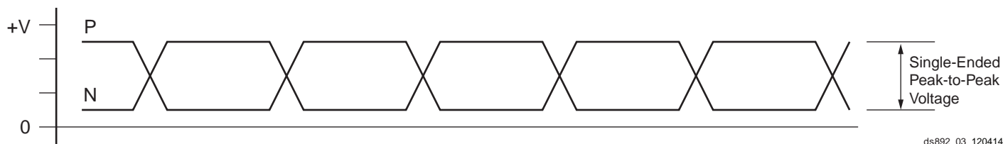
図 1: シングルエンドの電圧幅
