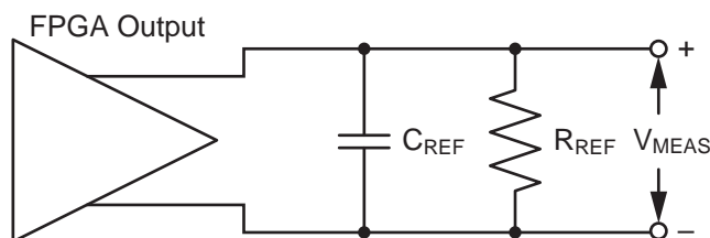
図 1: 差動のテスト セットアップ
