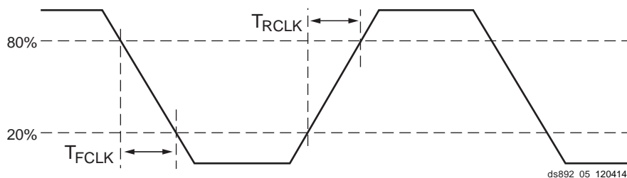
図 1: 基準クロックのタイミングパラメーター
