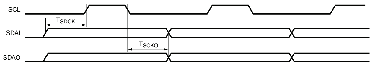
図 1: 標準モードの I2C インターフェイスのタイミング図
