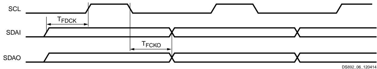
図 1: 高速モードの I2C インターフェイスのタイミング図
